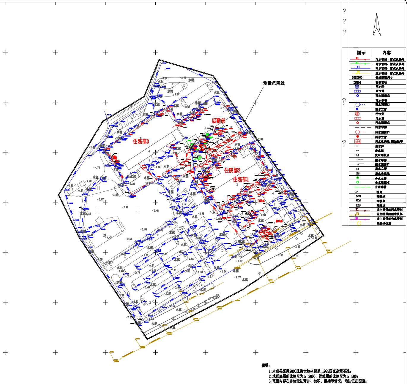
排水管线探测成果图-珠海市第五人民医院
